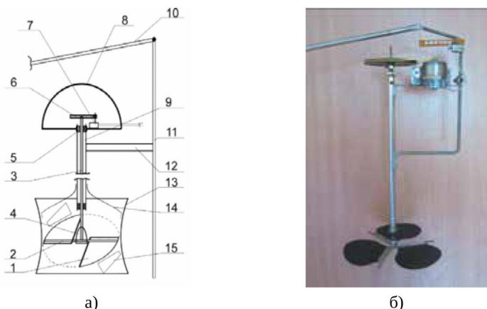
Рис. 2.19. Хвильова енергетична установка з гнучкими лопатями: а) схема; б) діюча модель
