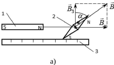
Рис. 2.12. Схема (а) та діюча модель (б) пристрою для вимірювання індукції магнітного поля постійного магніту:
